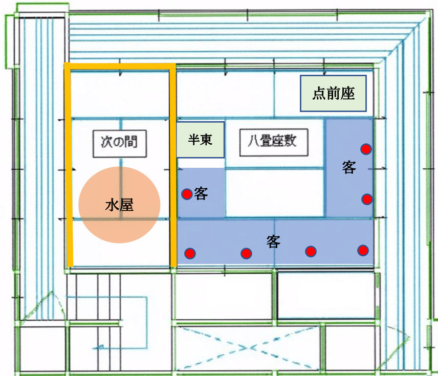
母屋二階平面図
